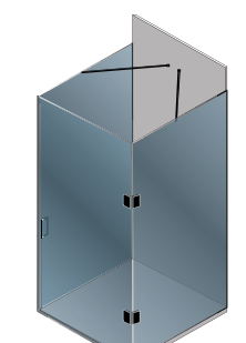
KIT E - VETRO / VETRO KIT E - GLASS / GLASS
