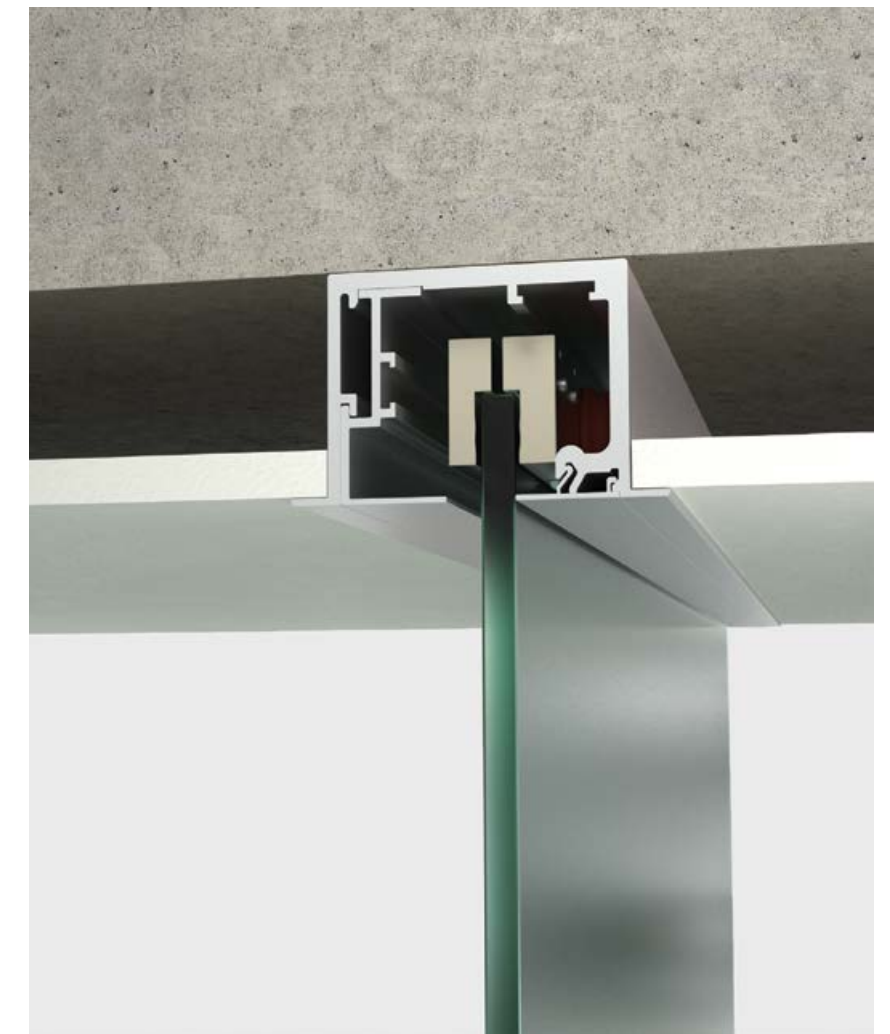
Porta scorrevole con binario Filomuro Wall Sliding door with Filomuro Wall track Porte coulissante avec rail Filomuro Wall Puerta deslizante con rail Filomuro Wall Schiebetür mit Schiene Filomuro Wall Раздвижная дверь с направляющей типа Filomuro Wall
